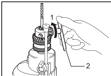
► 1. Tighten 2. Chuck key
