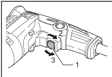
► 1. Vis de réglage de vitesse 2. Plus rapide 3. Abaisser
