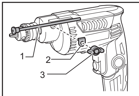
► 1. Jauge de profondeur 2. Rondelle 3. Vis de serrage
