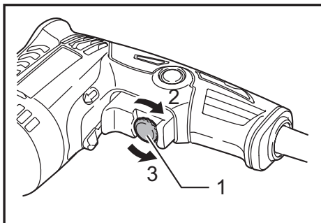
► 1. Disco de control de velocidad 2. Alta 3. Baja
