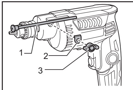
► 1. Calibrador de profundidad 2. Arandela 3. Tornillo de fijación
