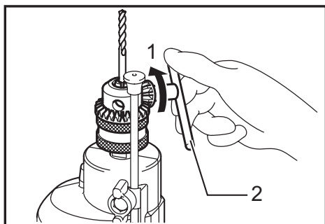
► 1. Serrer 2. Clé de mandrin
